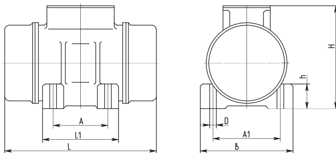
Рисунок 2. Вибраторы ЭП 99/220
